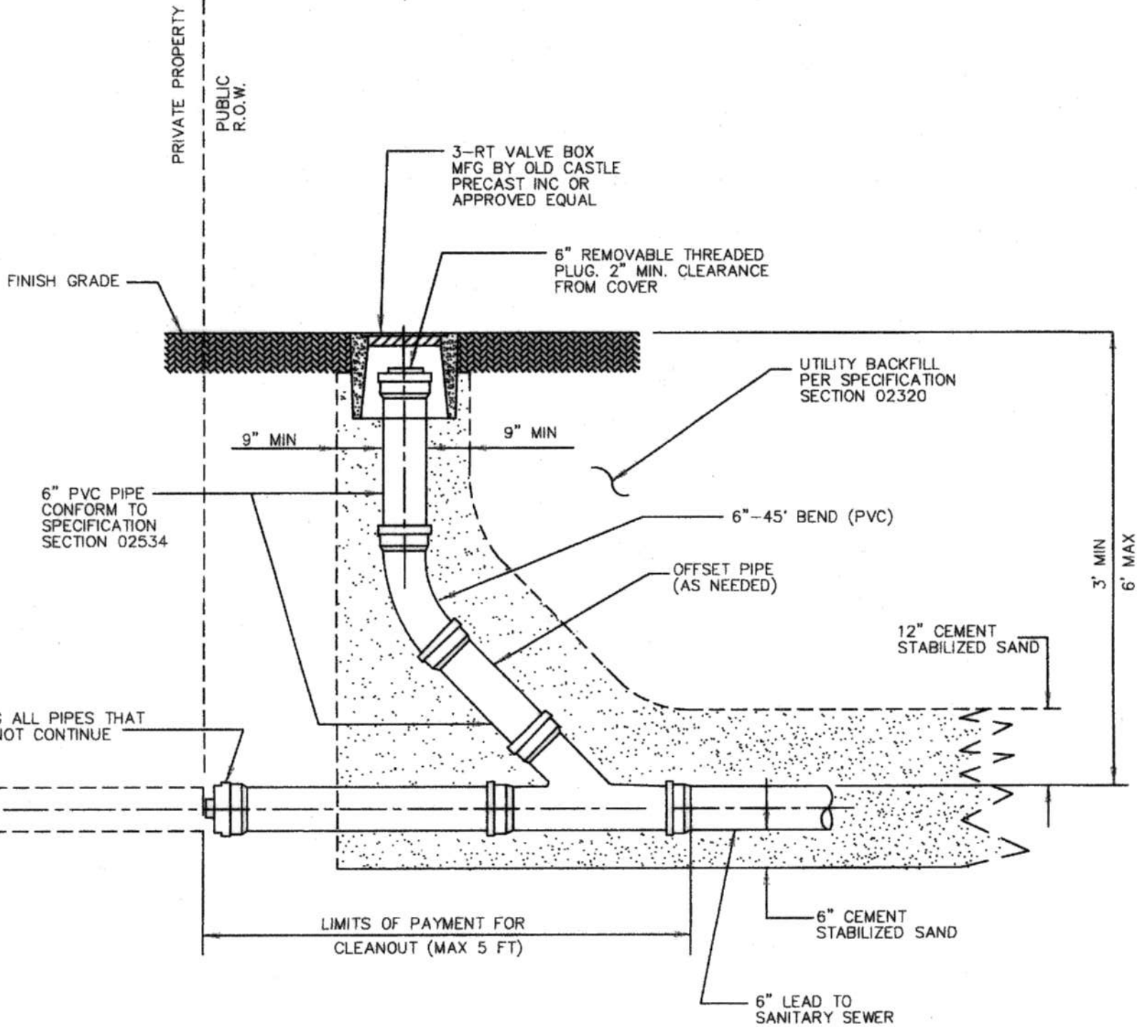
SECTION A-A
